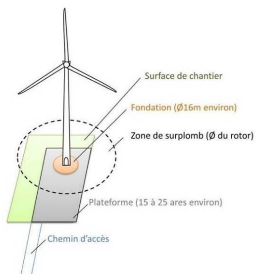
Illustration des emprises au sol d'une éolienne
