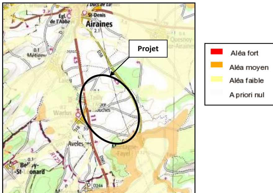
Carte du zonage du retrait-gonflement des argiles
